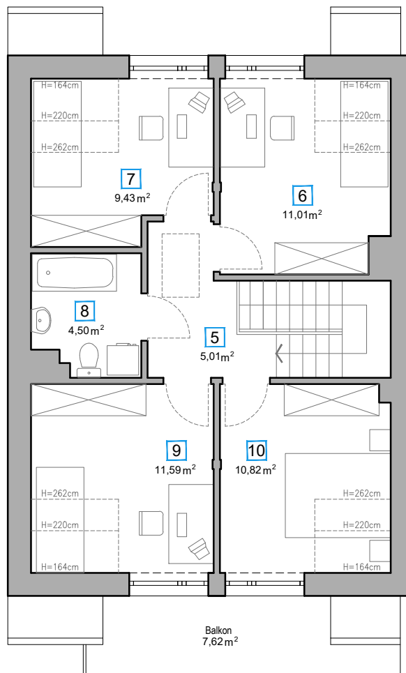
RZUT PODDASZA
