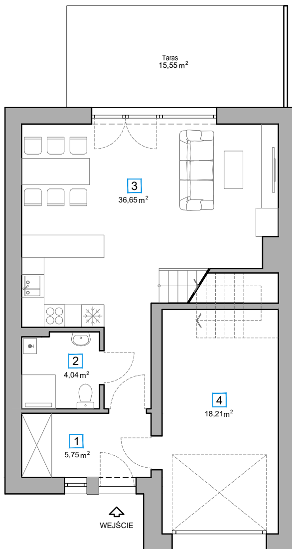
RZUT PARTERU
