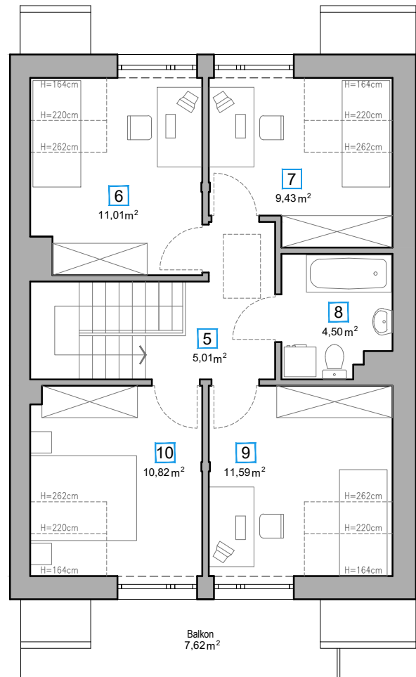
RZUT PODDASZA
